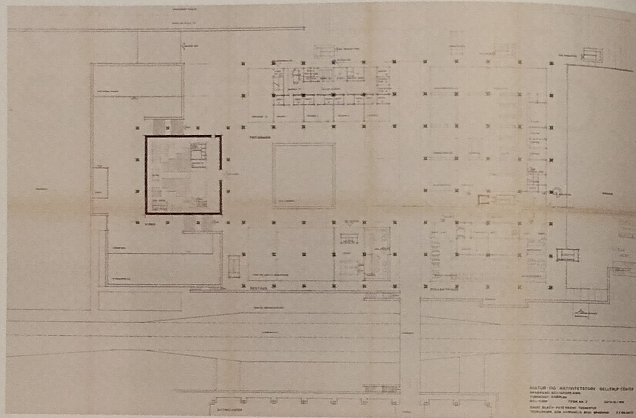
Kultur- og aktivitetstov, Gellerup. Stueplan. Tegning: Knud Blach Petersens Tegnestue
